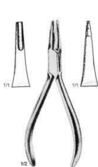
MSI-1981-13 Tweed 13.5 cm
